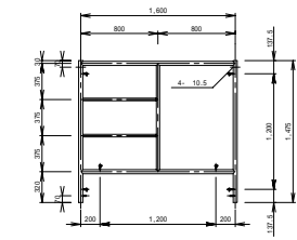
AB1615U (先メッキ) AB1615M (ドブメッキ)
