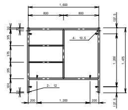
AB1615SUH (先メッキ) AB1615SH (ドブメッキ)
