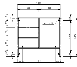
AB1615FU (先メッキ) AB1615FM (ドブメッキ)
