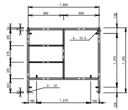
AB1615FUH (先メッキ) AB1615FHH (ドブメッキ)
