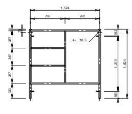
AB1515FU (先メッキ) AB1515FM (ドブメッキ)
