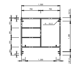
AB1515U (先メッキ) AB1515M (ドブメッキ)
