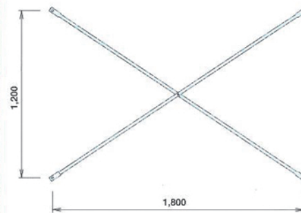
筋かい：BX1812
